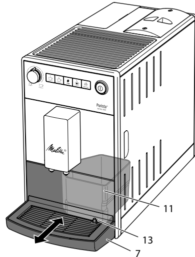
Abb. 8: Tropfschale und Kaffeessatzbehälter entleeren
